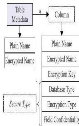
Fig.3. Structure of table metadata.
