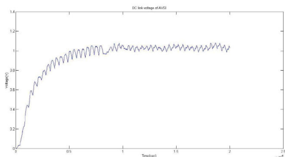
Fig.7 DC-link voltage of AVSI.
